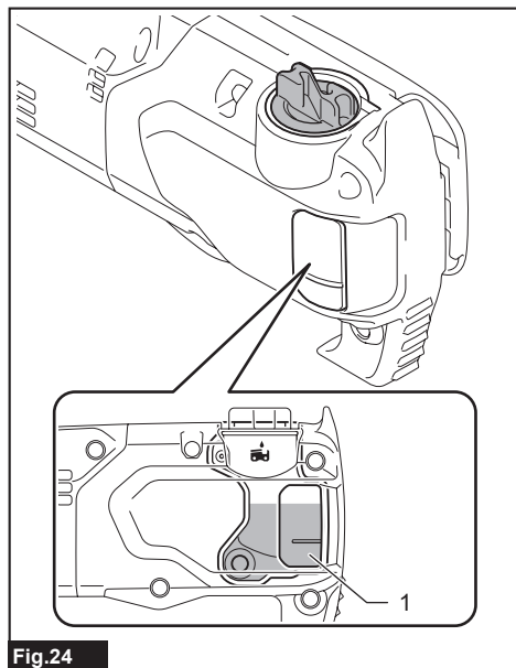
► 1. Réservoir d'huile
