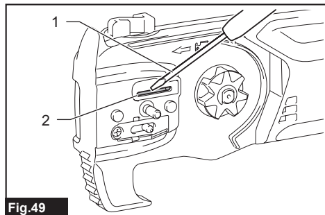
Fig. 49 ► 1. Tournevis plat 2. Orifice de vidange d'huile
