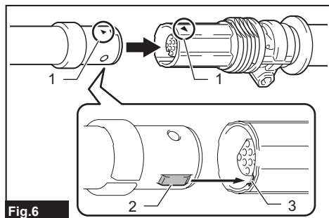
► 1. Marque triangulaire 2. Languette 3. Rainure
