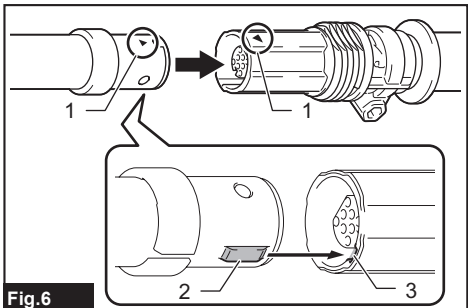
Fig.6 ► 1. Triangle mark 2. Tongue 3. Groove
