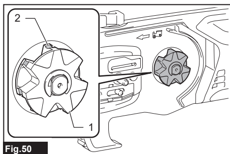
Fig. 50 ► 1. Pignon 2. Zones qui s'usent
