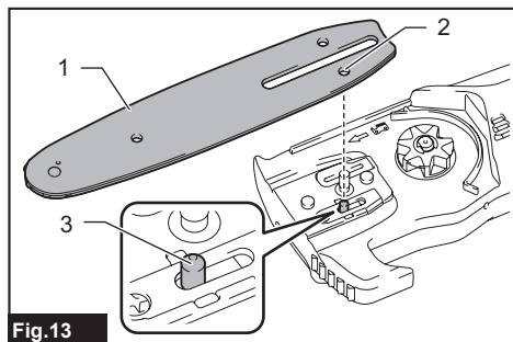
► 1. Barra de guía 2. Orificio 3. Pasador
