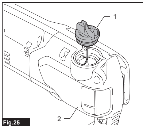
► 1. Bouchon du réservoir d'huile 2. Réservoir d'huile (translucide)
